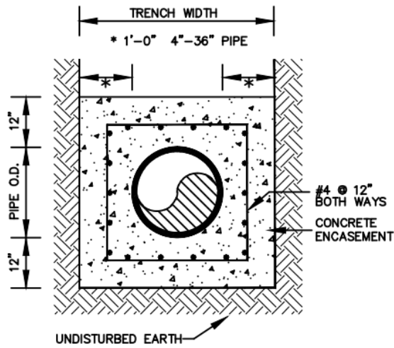
REINFORCED CONCRETE ENCASEMENT N.T.S.
