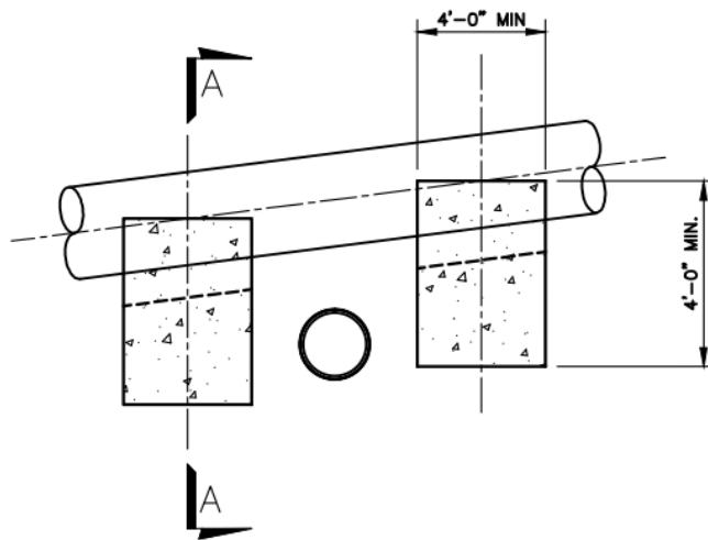
CONCRETE PEDESTAL N.T.S.
